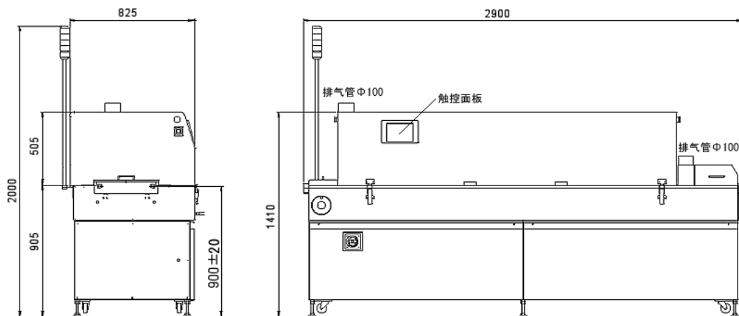
外形尺寸图
